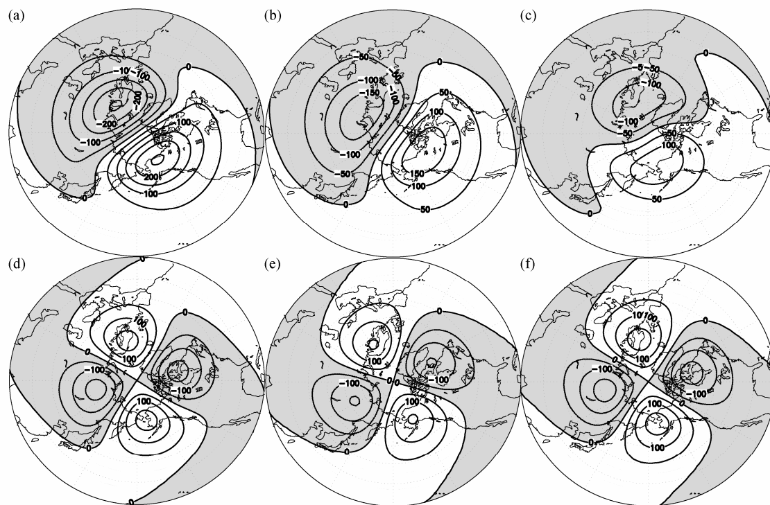
图 3 北半球冬季 12~2 月 100~20 hPa 位势高度场谐波分析 (a、b、c) 1 波和 (d、e、f) 2 波分布: (a, d) NCEP; (b, e) SAMIL; (c, f) BCC_AGCM。阴影: 小于 0 区域
