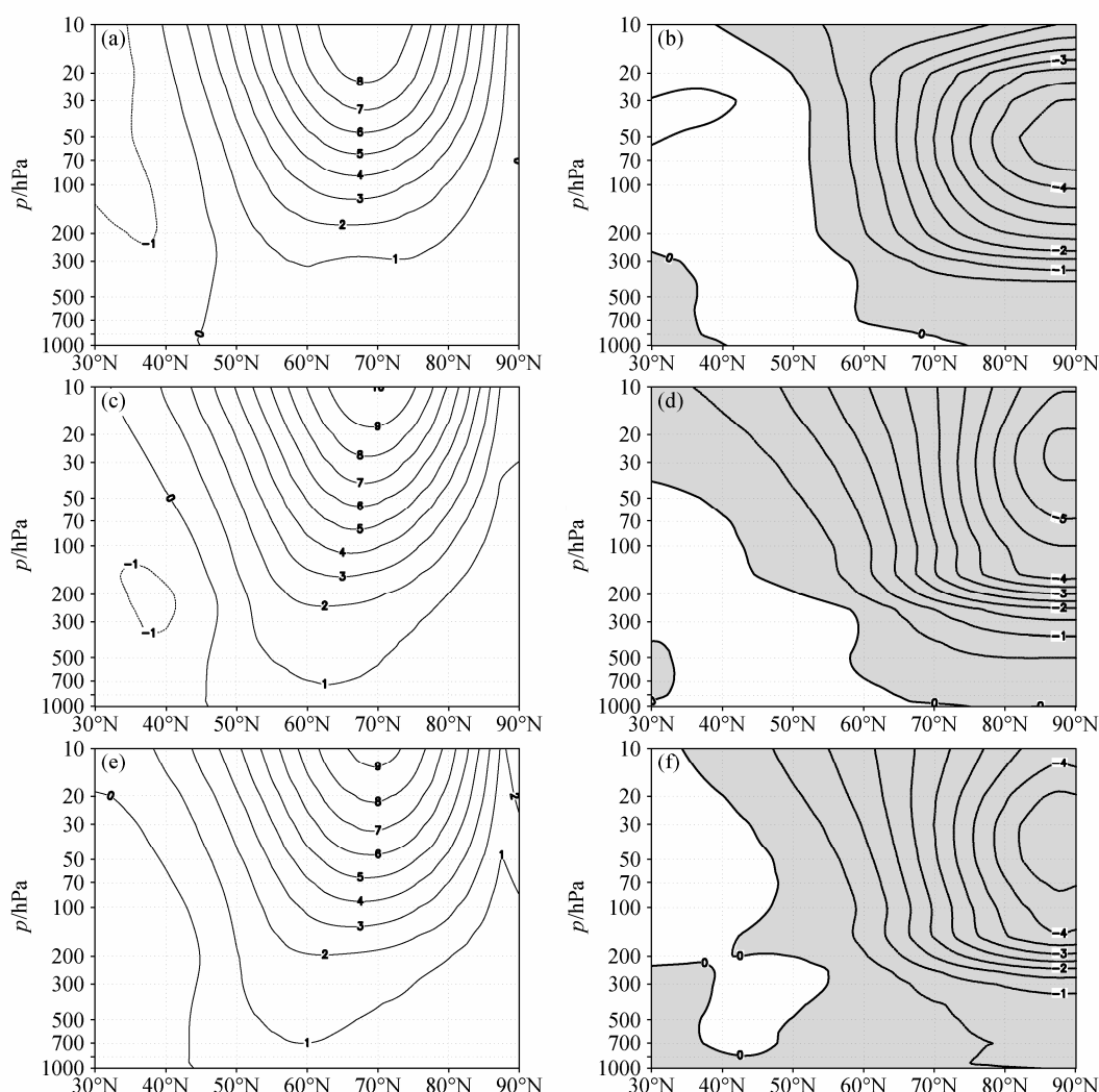
图7 纬向平均纬向风异常场 EOF 第一模空间分布 (a、c、e) 和用相应第一模态时间序列回归的纬向平均温度异常场的分布 (b、d、f, 单位: K): (a、b) NCEP; (c、d) SAMIL; (e、f) BCC_AGCM. 阴影: 负异常区域
