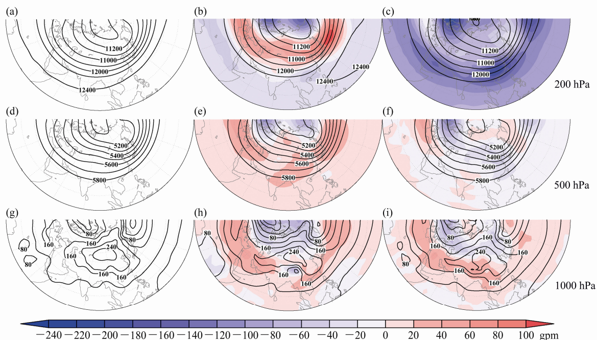
图4 北半球冬季12~2月气候平均的200 hPa、500 hPa和1000 hPa高度场分布(单位: gpm): (a、d、g) NCEP; (b、e、h) SAMIL; (c、f、i) BCC_AGCM。阴影: 相应的模式与NCEP之间的差值
