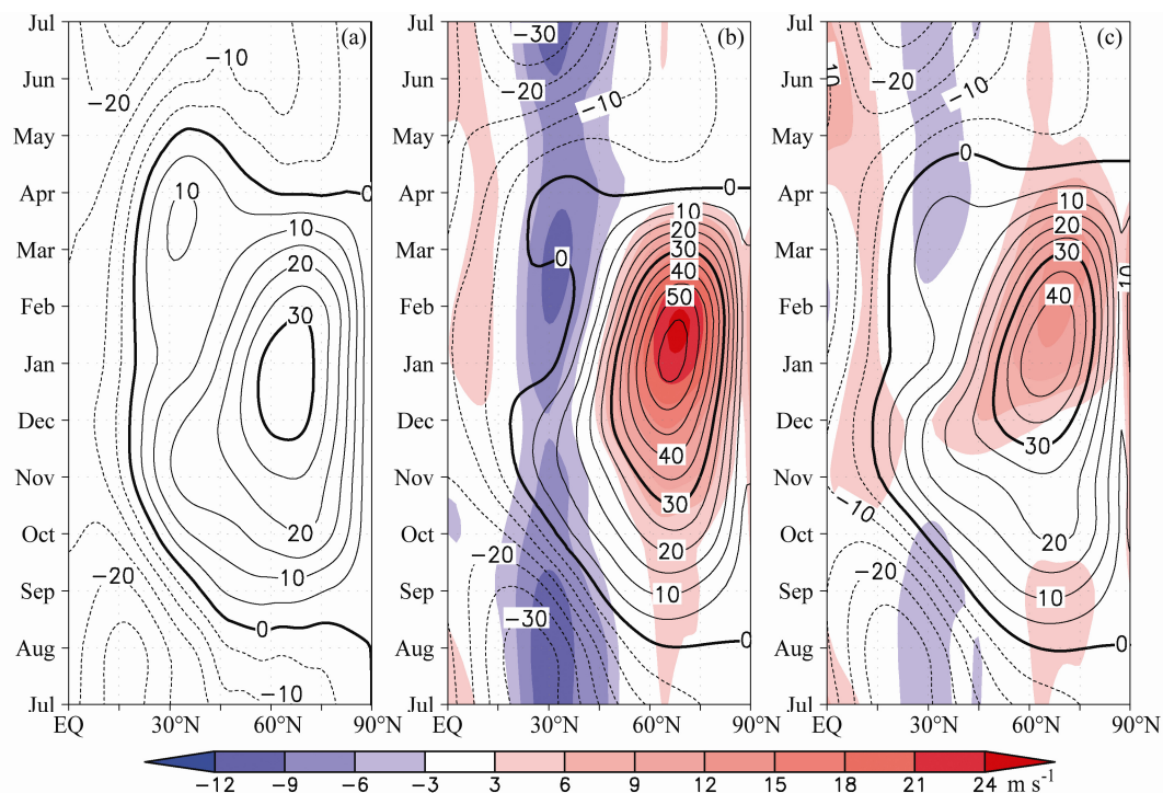
图 5 北半球气候平均 10 hPa 纬向平均纬向风 (单位: \text{m/s} ) 的年循环分布: (a) NCEP; (b) SAMIL; (c) BCC_AGCM。阴影: 相应的模式与 NCEP 的偏差
