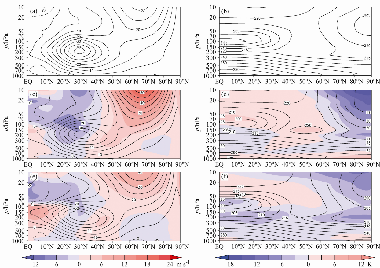
图 1 北半球冬季 12~2 月气候平均的纬向平均纬向风 (a、c、e, 单位: \text{m/s} ) 和纬向平均温度 (b、d、f, 单位: \text{K} ) 分布: (a) NCEP 纬向平均纬向风场; (b) NCEP 纬向平均温度场; (c) SAMIL; (d) SAMIL; (e) BCC_AGCM; (f) BCC_AGCM. (c-f) 阴影: 相应模式与 NCEP 场的差值
