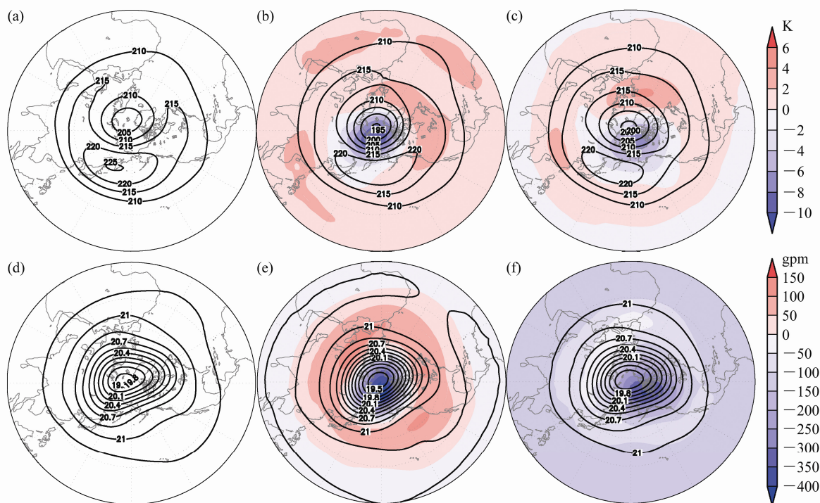
图2 北半球冬季12~2月气候平均的100~20 hPa温度场(a、b、c, 单位: K)以及位势高度场(d、e、f, 线条单位: gpm; 彩色阴影单位: gpm)分布: (a) NCEP; (b) SAMIL; (c) BCC_AGCM; (d) NCEP; (e) SAMIL; (f) BCC_AGCM。阴影: 相应模式与NCEP场的差值
