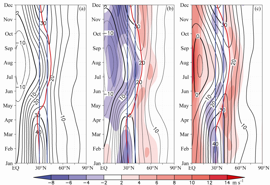
图 6 北半球气候平均 200 hPa 纬向平均纬向风 (单位: \text{m/s} ) 的年循环分布: (a) NCEP; (b) SAMIL; (c) BCC_AGCM。蓝线: 30°N 和 40°N 位置; 红线: 副热带西风急流轴; 阴影: 相应模式与 NCEP 的差值
