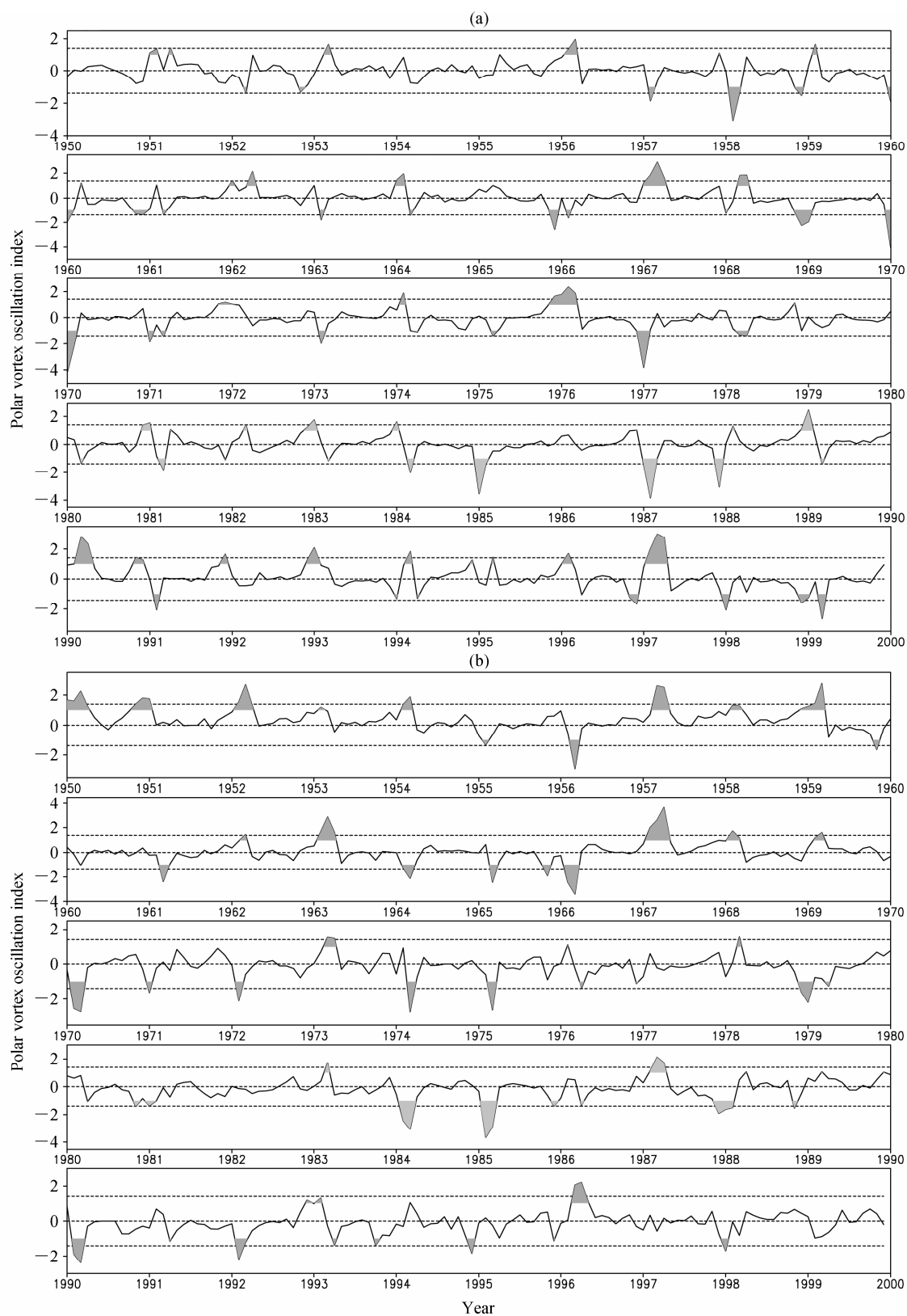
图9 极涡振荡指数分布: (a) NCEP; (b) SAMIL; (c) BCC_AGCM。虚线: 1.4个标准差; 阴影: 大于1个标准差的量值
